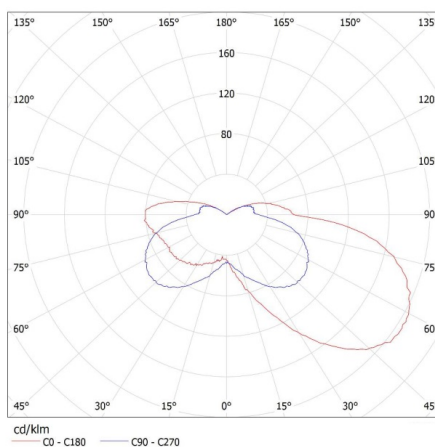
KANLUX S.A. (kat 23802) SABIK LED AC-WW / LDC (Polar)
